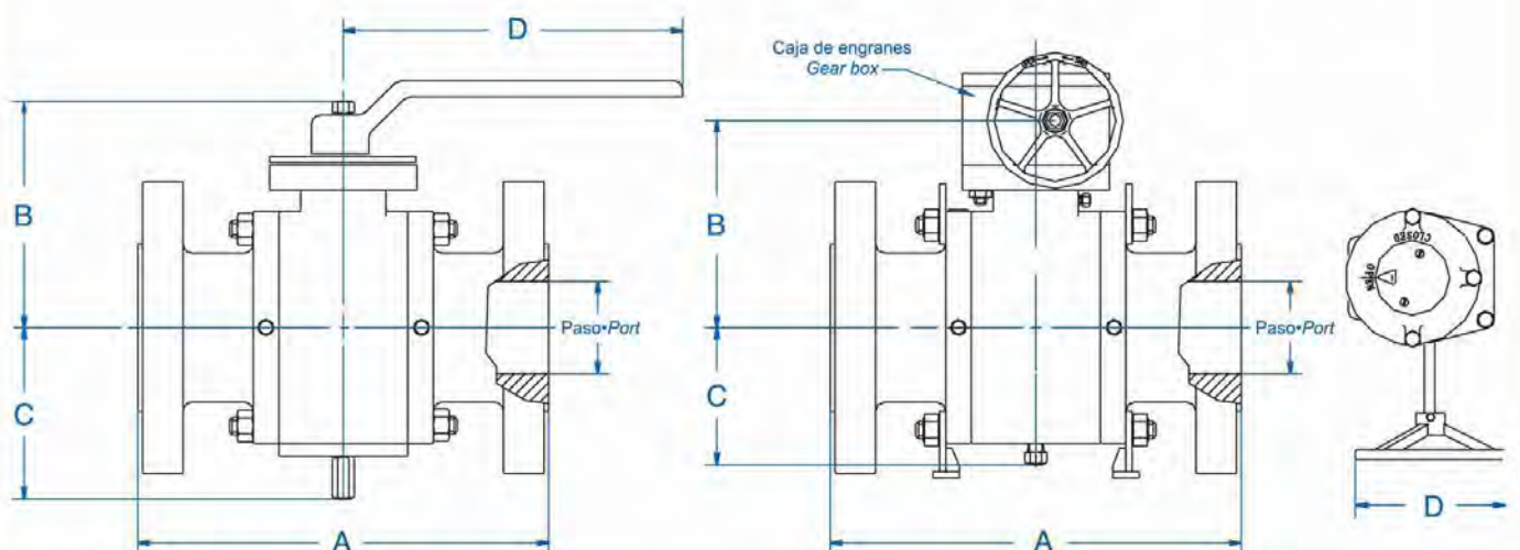
Dimensiones • Dimensions
