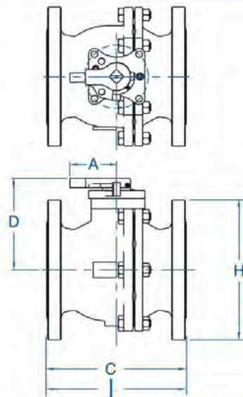
Serie F-152 A Prueba de Fuego • Series F-152 Fire Safe
