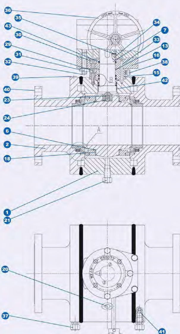
Lista de partes para válvulas de cuerpo integral Soldado List of components for welded valves
