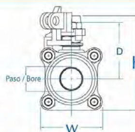
Dimensiones • Dimensions
