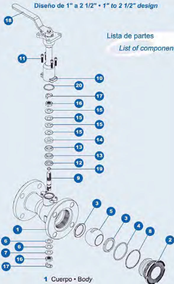
Diseño de 1" a 2 1/2" • 1" to 2 1/2" design
