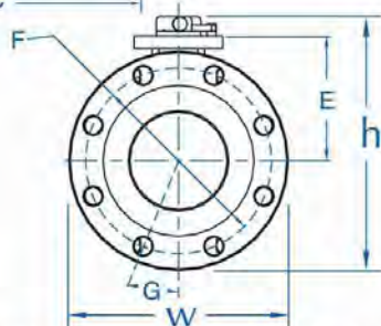
Serie F-152 A Prueba de Fuego • Series F-152 Fire Safe
