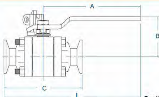
Dimensiones • Dimensions
